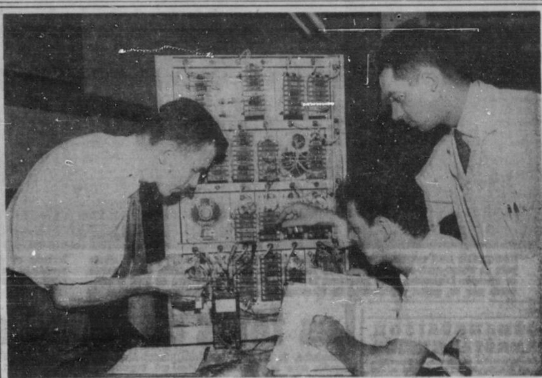
A L'INSTITUT TECCART, l'enseignement des circuits électroniques avancés se fait à l'aide d'un système de démonstration des plus perfectionnés. A son tour, l'étudiant peut répéter l'expérience au laboratoire en utilisant des montages tels que ceux rencontrés dans l'industrie. La photo montre deux professeurs préparant une expérience qui sera ensuite faite par les étudiants.
