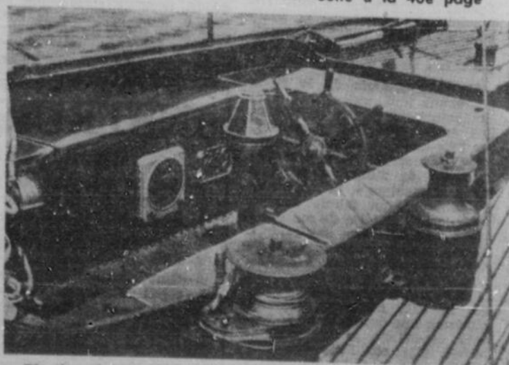
Fig. 4 — Le winches, ces treuils à tambour aidant le réglage des drisses et des écoutes, sont surtout nécessaires pour les gros efforts. Il s'en fait de petits modèles pour le yachting léger. (Photo Yachting)
