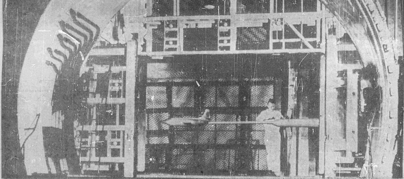
Un modèle apprêté pour l'essai. — Un technicien met le dernier touché à l'ajustement d'un modèle qui subira bientôt les furies d'un vent d'une vélocité qui dépasse de 1.3 la vitesse du son. L'air frappe l'appareil tout comme s'il était dans le ciel mais à une vitesse de beaucoup supérieure.
