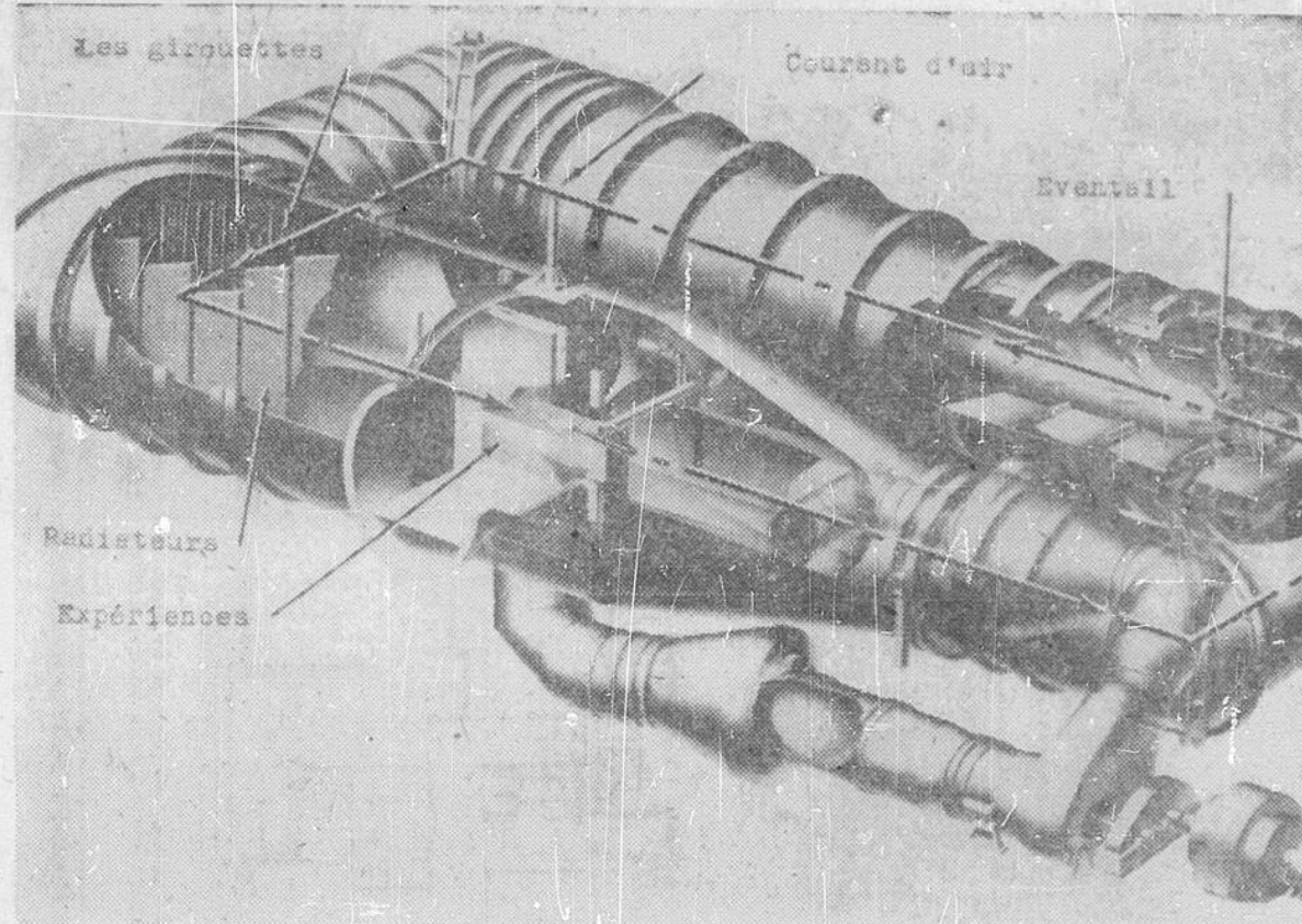
Voici une coupe du fameux tunnel à air des laboratoires électroniques Cornell où se font la majorité des essais avant la fabrication des avions. Dans ce tunnel on peut développer des vents d'une vélocité de 1,000 milles à l'heure. Deux moteurs de 22,000 chevaux-vapeur actionnent des ailes d'éventail et poussent l'air dans un tunnel. L'air pénètre dans la salle d'essai par un débouché restreint, ce qui augmente la pression.
