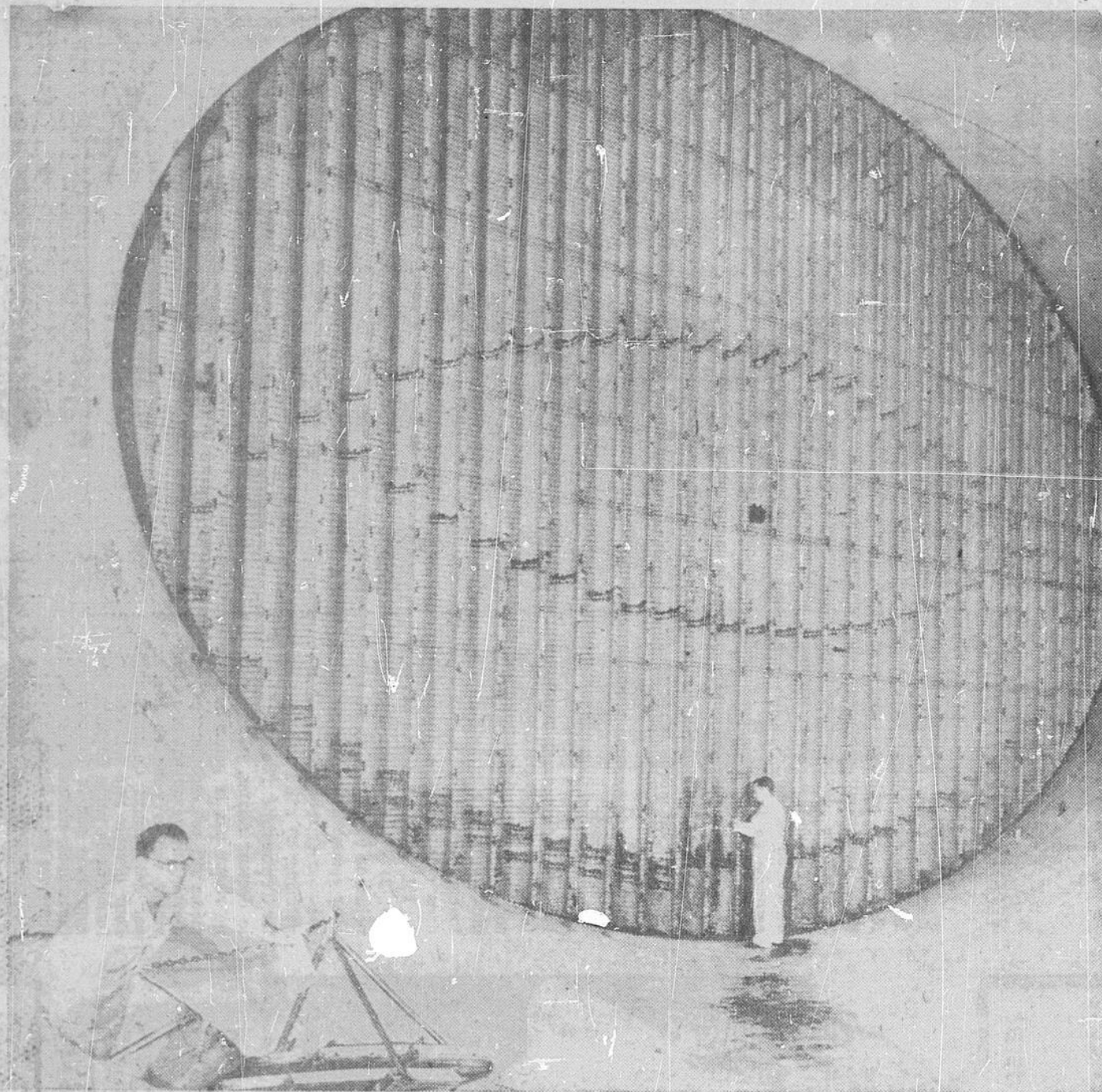
Pour détourner le courant d'air. — Ces immenses ailettes servent à diriger gentiment le courant d'air dans le premier tournant du tunnel à air. A cet endroit précis, le tunnel a un diamètre de 32 pieds.
