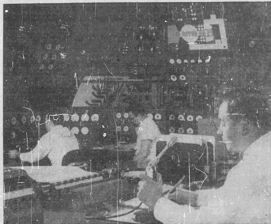
La salle de contrôle. — C'est ici que réside le centre de toutes les opérations d'un essai. Ce qui se passe dans le tunnel à air et sur le modèle à l'essai est entièrement enregistré et contrôlé par des instruments à distance. Des instruments de calcul dans la salle de contrôle servent à enregistrer et analyser les réactions du modèle à l'essai.
