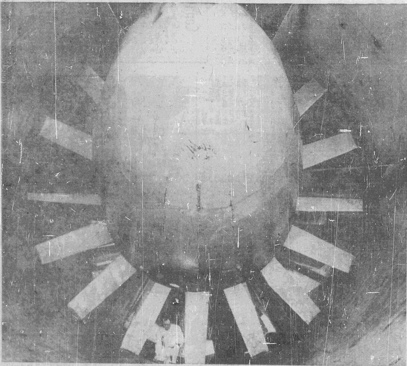
Les ailes du troisième éventail. — La photo ci-haut nous montre les ailes immenses du troisième et dernier éventail qui se trouve dans le tunnel à air. Pour régler la vitesse de l'air dans le tunnel, on contrôle l'angle de disposition des ailes sur l'éventail. Chacune de ses ailes pèse 275 livres.
