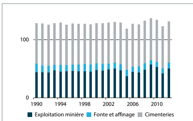
GRAPHIQUE 9 - Intensité en GES pour certains secteurs en lien avec le secteur minier au Québec, 1990-2012 (tonnes/TJ)
