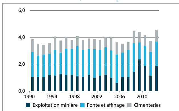
GRAPHIQUE 8 - Émissions de GES de secteurs en lien avec le secteur minier au Québec, 1990-2012 (en millions de tonnes équivalent CO 2 )
