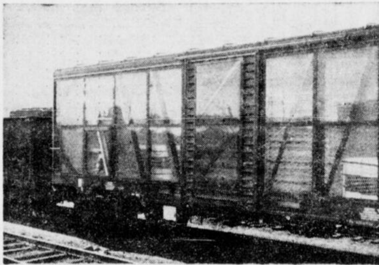
UN WAGON-MARCHANDISES UNIQUE EN SON GENRE vient d'être construit par le Canadien National pour renseigner ses employés et ses clients sur les meilleures méthodes de chargement et de manutention des marchandises. Ce wagon comporte une paroi en plexiglas qui permettra de se rendre compte du résultat d'un chargement, d'un accouplement ou d'un emballage impropres. (Photo Canadien National)
