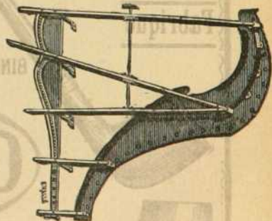
Barres de fer forgé pour pianos à queue Poids 52 Kgs.
