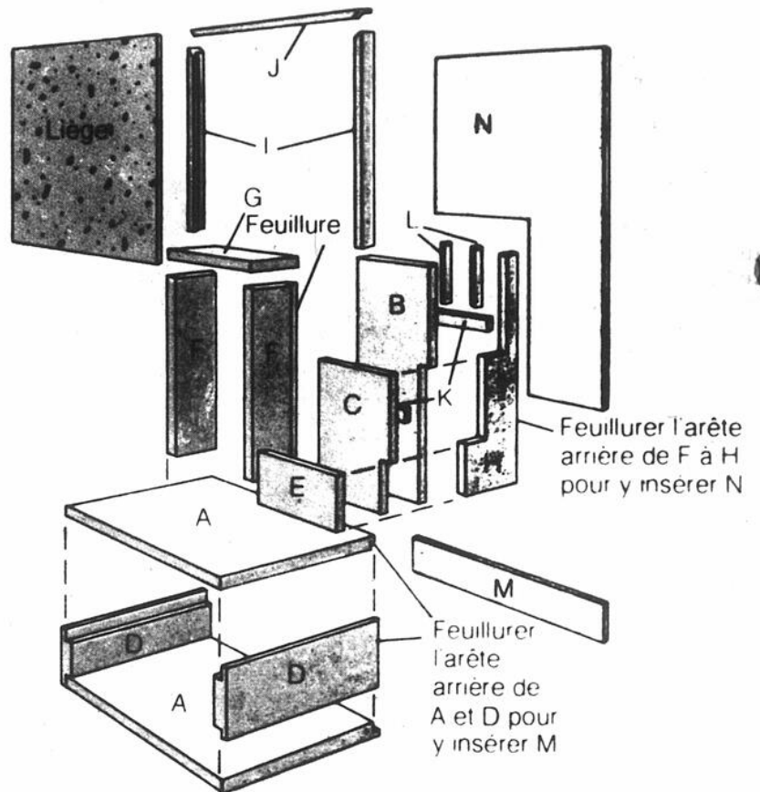
Dimensions hors tout Longueur = 16 pouces
