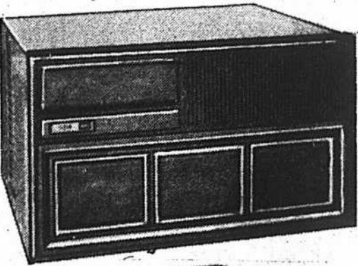
Modèle à puissance 11,000 BTU, moteur 115 volts 12 ampères. Grilles d'évacuation d'air réglables.
