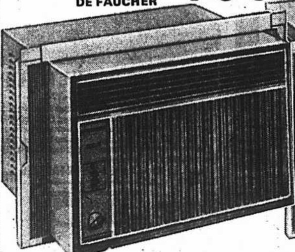
Modèle ARB100-2 — Puissance 10,000 BTU. Moteur 115 volts, 12 ampères. Agit sur 700 pieds carrés.
