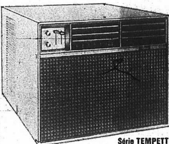
Série TEMPETTE Puissance 5000 BTU, moteur 115V, 7.5 amp. Puissance 6000 BTU, moteur 115V, 10.7 amp. Puissance 8000 BTU, moteur 115V, 12 amp.
