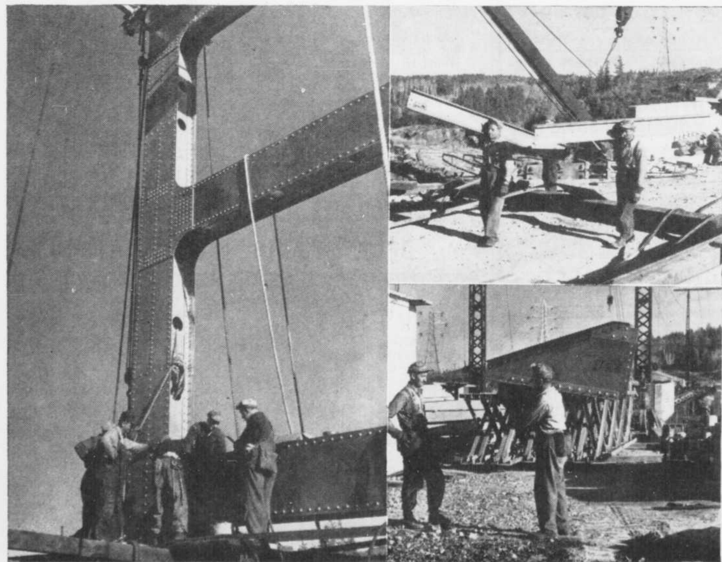
A gauche: On boulonne l'une des poutres transversales des piliers principaux. A gauche, en haut: Deux employés, MM. Almas Desbiens et René Lavoie transportent des poutrelles en aluminium. Le poids de ces pièces est de 96 livres alors qu'il serait d'environ 309 livres si elles étaient en acier; en bas, M. Almas Desbiens porte aisément une pièce, d'aluminium de 140 livres; la même pièce, en acier, pèserait 420 livres.
