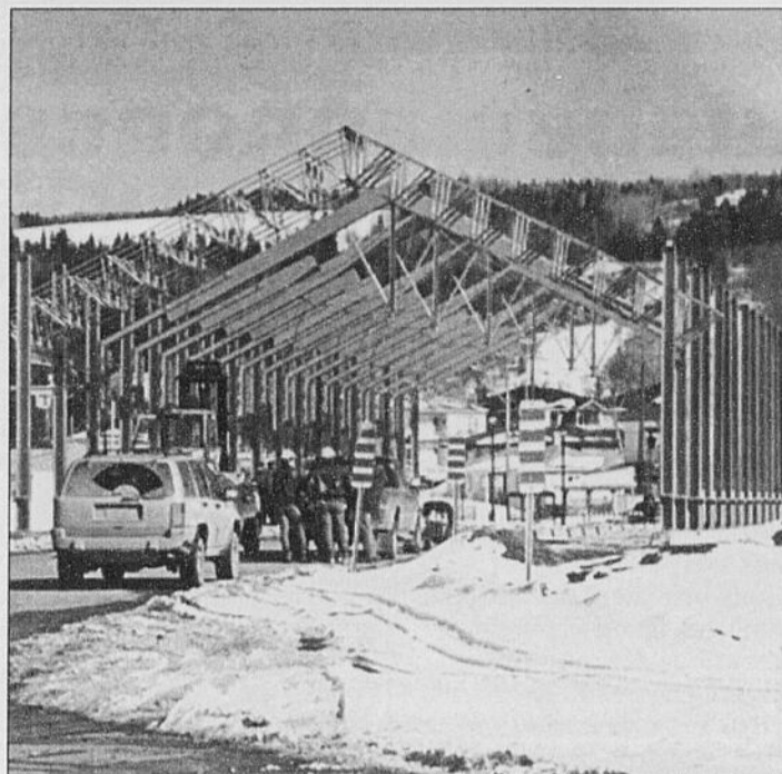
STRUCTURE - Le nouveau pont urbain du secteur Saint-Alexis à La Baie est maintenant doté d'une structure en acier galvanisé qui donne l'illusion d'un pont couvert.
