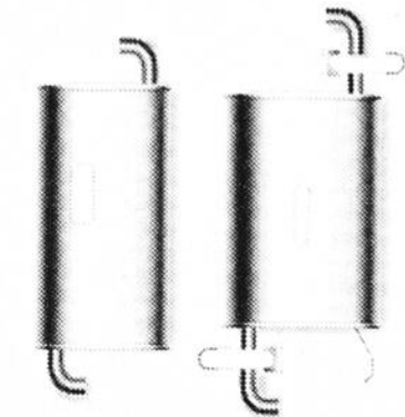
CHEZ HONDA SILENCIEUX MONOPIECE CHEZ UN CONCURRENT SILENCIEUX MULTIPIECES
