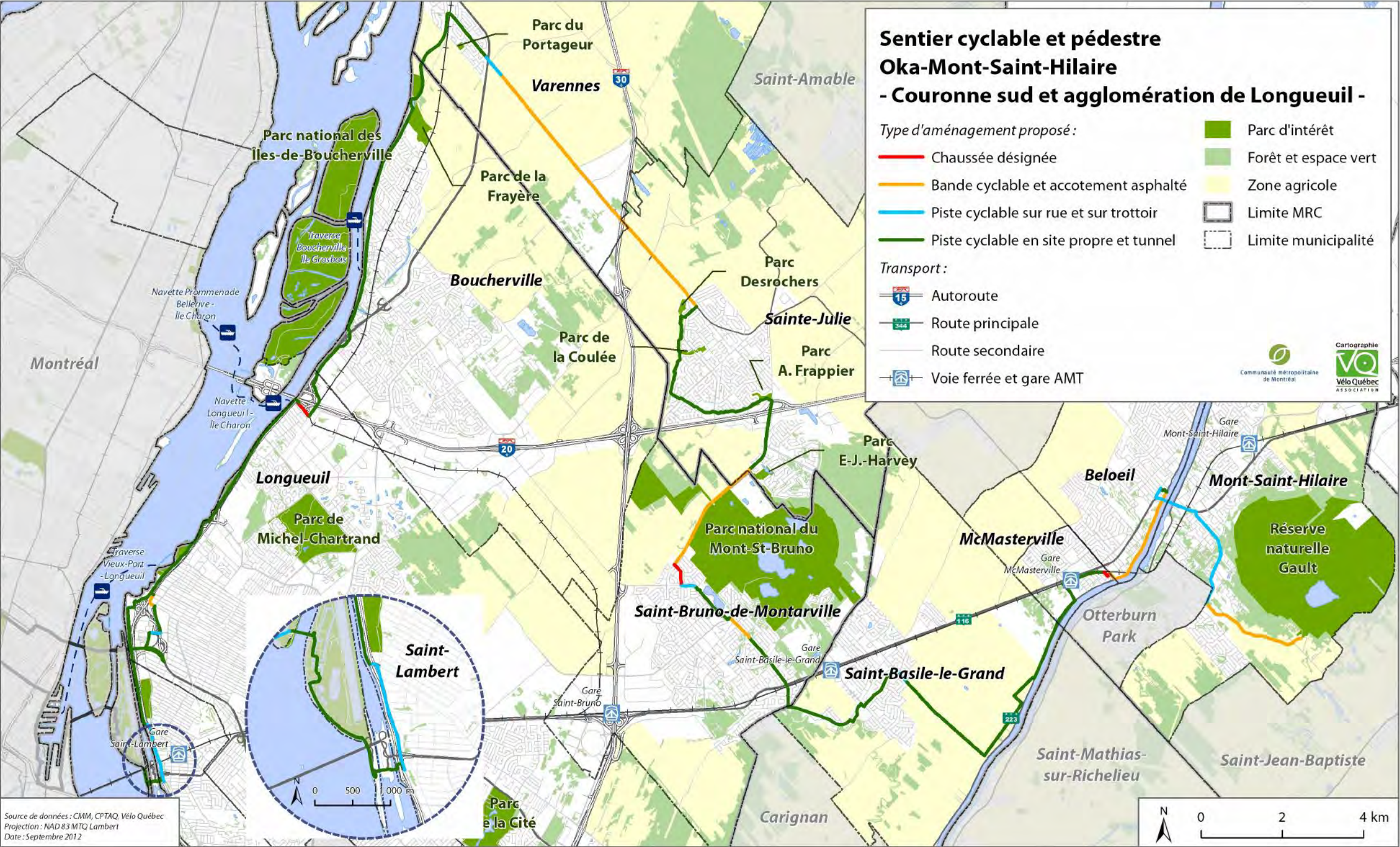
Carte 6. Agglomération de Longueuil et couronne Sud – aménagements proposés sur le tracé recommandé
