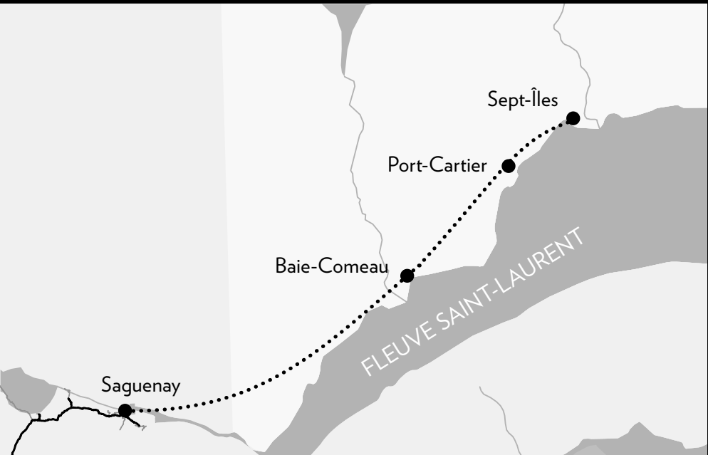
Un tuyau d'acier de 16 pouces de diamètre sera enfoui à 1 mètre dans le sol sur une distance de 450 kilomètres.
