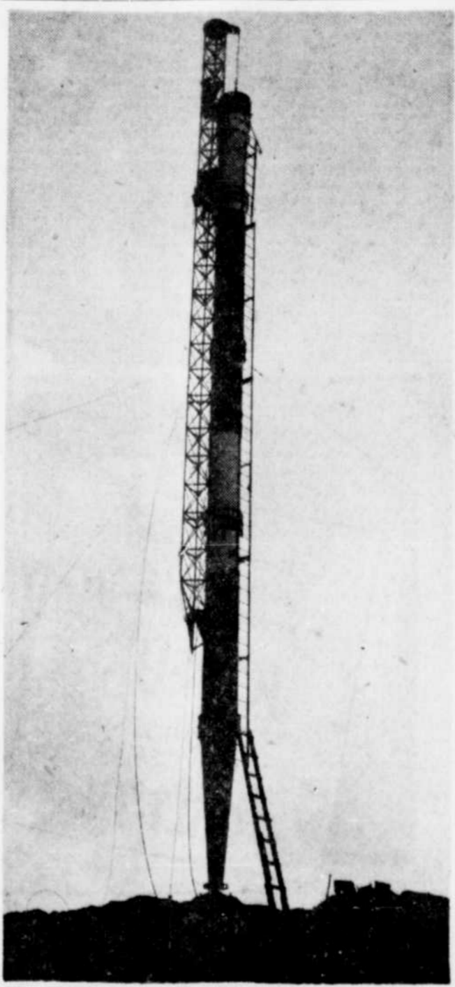
Cette antenne cylindrique de CHLT-TV, canal 7, sur le mont Orford atteint une hauteur de 150 pieds. Elle transmet les images et les sons produits dans les studios du poste de La Tribune.
