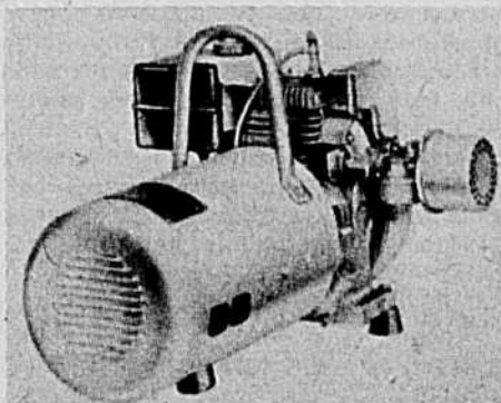
Alternateur WINPOWER: Maska Auto Electric, distributeur de Winpower Corp.,
