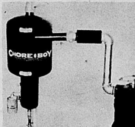
Récupérateur d'huile, filtre et silencieux: Le tout nouveau récupérateur d'huile et silencieux CHORE-BOY est de type monobloc sans aucune partie mobile et,
