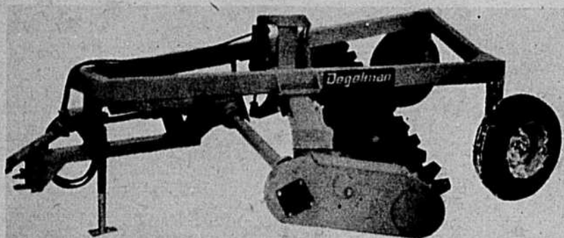
RÂTEAU À ROCHES DEGELMAN Met les roches de 2" à 36" de dia., en andain. Largeur de travail: 14'.
