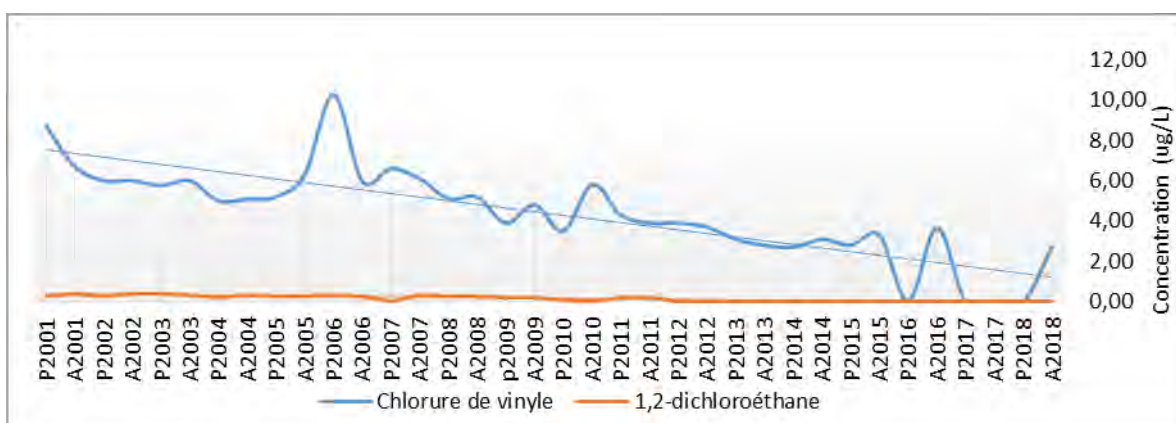
GRAPHIQUE 11. ÉVOLUTION DES CONCENTRATIONS DE CHLORURE DE VINYLE ET DE 1,2-DICHLOROÉTHANE DANS LE PUIT D'OBSERVATION PO-94-7R
