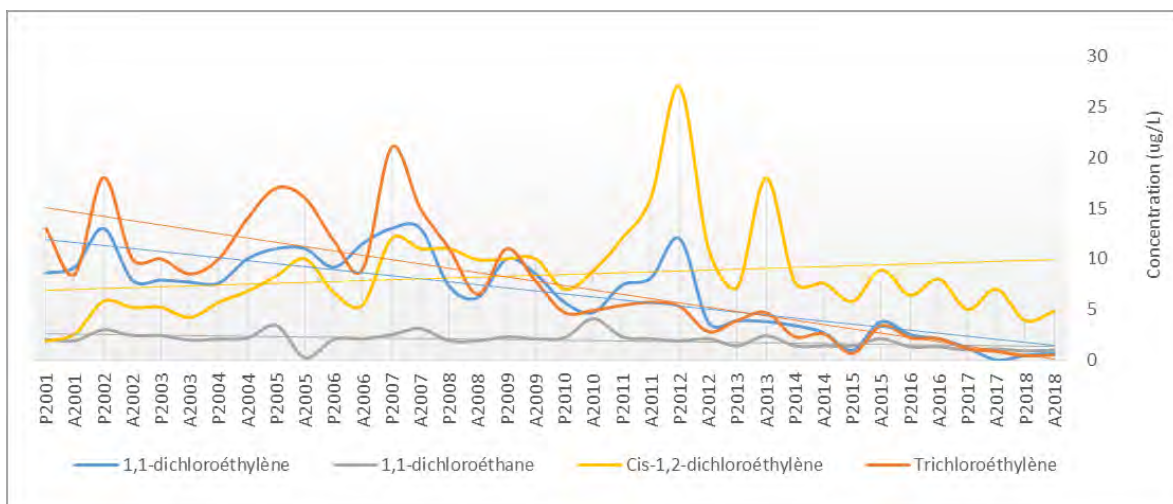
GRAPHIQUE 3. ÉVOLUTION DES CONCENTRATIONS EN 1,1-DICHLOROÉTHYLÈNE, 1,1-DICHLOROÉTHANE, CIS-1,2-DICHLOROÉTHYLÈNE ET TRICHLOROÉTHYLÈNE DANS LE PUIT D'OBSERVATION PO-94-1S
