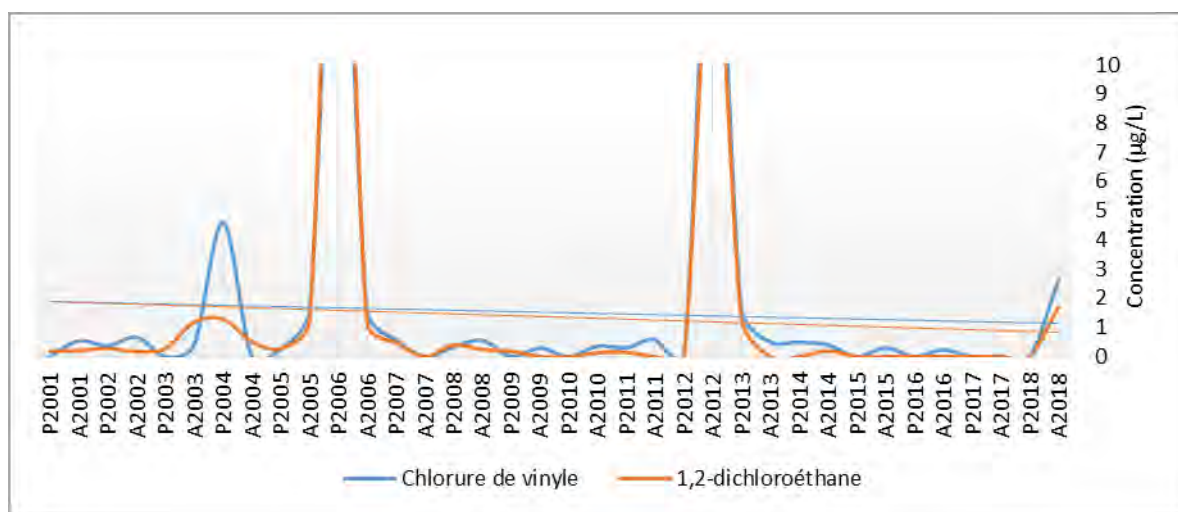
GRAPHIQUE 7. ÉVOLUTION DES CONCENTRATIONS EN CHLORURE DE VINYLE ET EN 1,2-DICHLOROÉTHANE DANS LE PUIT D'OBSERVATION 03097201
