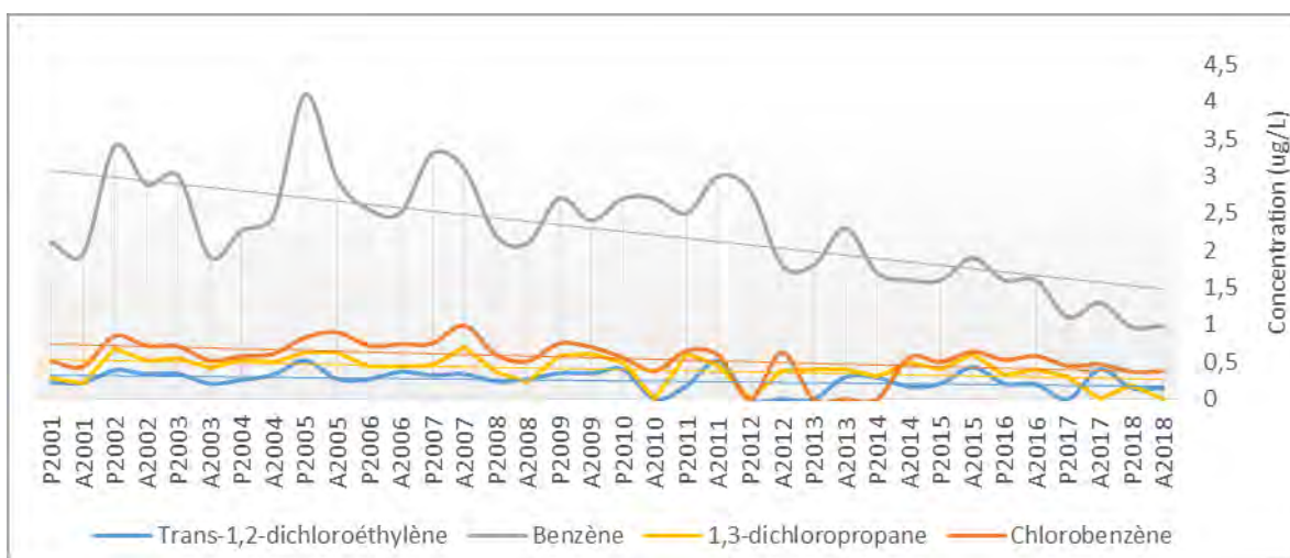
GRAPHIQUE 4. ÉVOLUTION DES CONCENTRATIONS EN TRANS-1,2-DICHLOROÉTHYLÈNE, BENZÈNE, 1,3-DICHLOROPROPANE ET CHLOROBENZÈNE DANS LE PUIT D'OBSERVATION PO-94-1S
