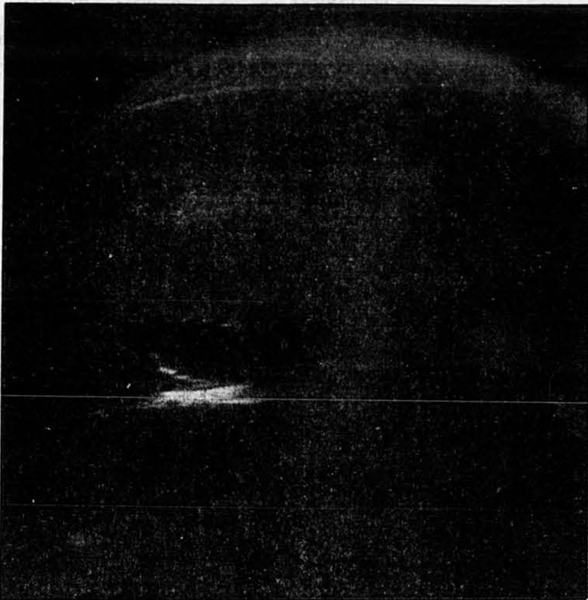
Voici Neptune, telle que Voyager 2 nous l'a fait découvrir cette semaine.
