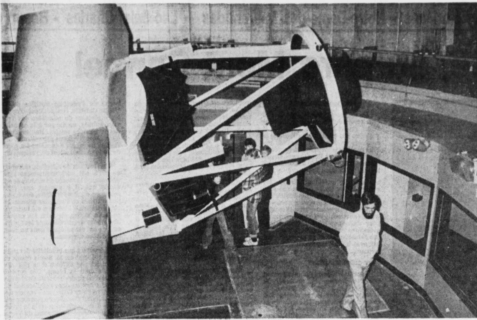
La coupole d'aluminium de 14 mètres de diamètre abrite le télescope de 22 tonnes.
