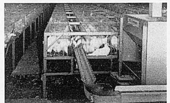
La moulée s'achemine sans cesse, et les pertes sont éliminées grâce aux trémies et à la chaîne d'alimentation Big Dutchman.
