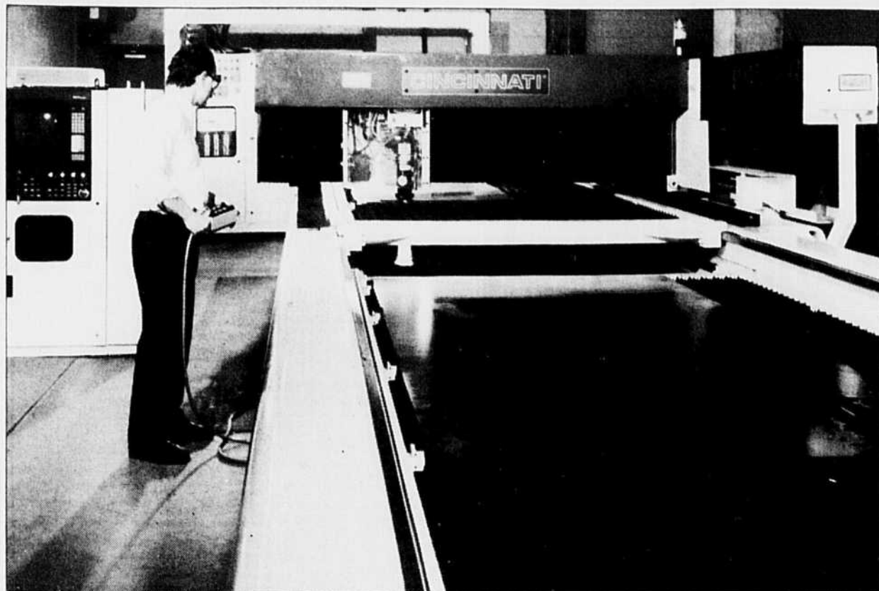
La dernière acquisition du CRIQ provient des USA. C'est une machine informatisée pour la coupe au laser de matériaux en feuilles (bois, plastic, métal).
