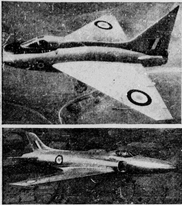
Les Anglais, pionniers de l'avion à réaction, redoublent leurs forces aériennes, déjà doublées, avec un programme de défense nationale de 13 milliards. Cette photographie nous montre les quatre plus récents modèles de chasseurs à réaction. Ce sont: en haut à gauche, le Boulton Paul P.111, dont les ailes rappellent la lettre grecque "D" (delta), avion d'essai. Les détails de son fonctionnement sont gardés secrets. En bas, à gauche, un avion d'essai, le Vickers Supermarine 535, mû par un moteur Rolls Royce; avec ses ailes rejetées en arrière, cet avion possède une vitesse exceptionnelle et peut monter à une très haute altitude. En haut à droite: le chasseur H.P. 88, construit par la Hendley Page et la Blackburn and General Aircraft, activé par un Rolls Royce. En bas, à droite, le De Havilland Sea Venom, mû par un moteur à turbine de Havilland Ghost. Muni du radar il transporte un équipage de deux hommes.
