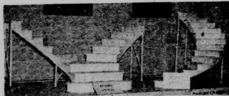
Ces escaliers, fabriqués par les élèves de 2e année à l'Ecole de menuiserie de l'Ecole Technique, semblent peut-être faciles à construire de prime abord. Leur réalisation est beaucoup plus difficile cependant. Le premier à gauche est un escalier à deux voies; l'autre est un cintre avec ébrasement irrégulier, c'est-à-dire que sa montée s'éloigne toujours de son rayon. Ces escaliers sont montés sur gabarits à segments parfaitement harmonisés. Les élèves inscrits à ces cours deviennent des techniciens du métier. Une foule d'objets sont actuellement exposés au public dans les différents ateliers de l'école. M. Poisson, du Bien-Être de la Jeunesse, a ouvert l'exposition en présence de M. Hector Beaupré, directeur de l'école, et de M. Joseph-Eudore Gamache, directeur de l'atelier de menuiserie.
