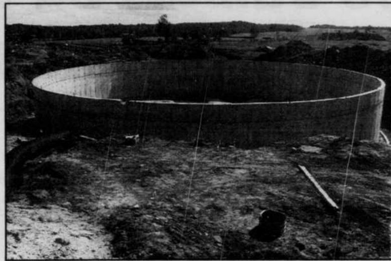
Yvan Ostiguy (à gauche) travaillait dans une tranchée (à droite) où il installait des tuyaux devant relier une fosse à purin (ci-dessus) à un champ d'épuration. Un amas de terre a glissé sur lui l'entraînant dans une mort affreuse.
