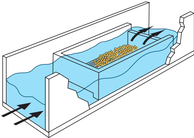
17. Incubateur de type californien (upwelling) (Anonyme, 1996)
