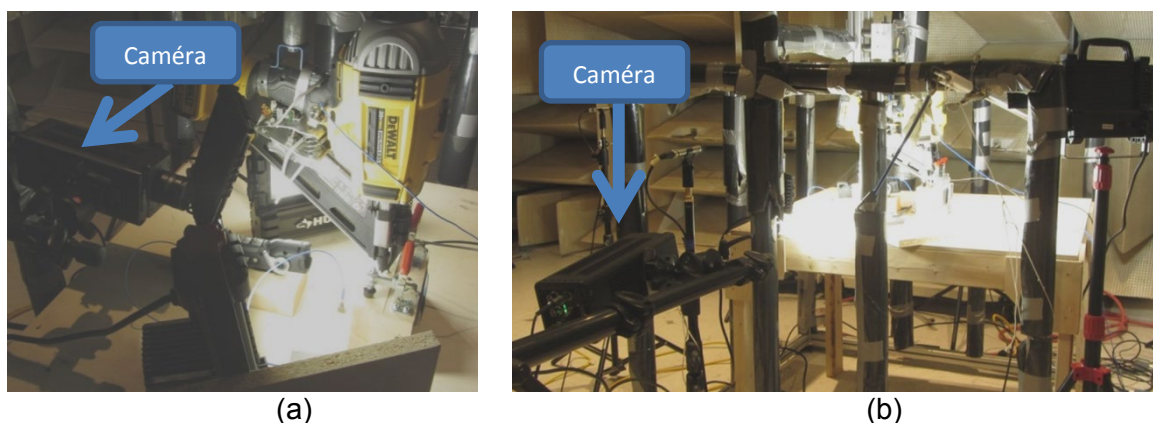
Figure 32 Caméra haute vitesse : (a) vue rapprochée pour mesurer l'enfoncement d'un clou et (b) vue éloignée pour mesurer le mouvement global de la cloueuse
