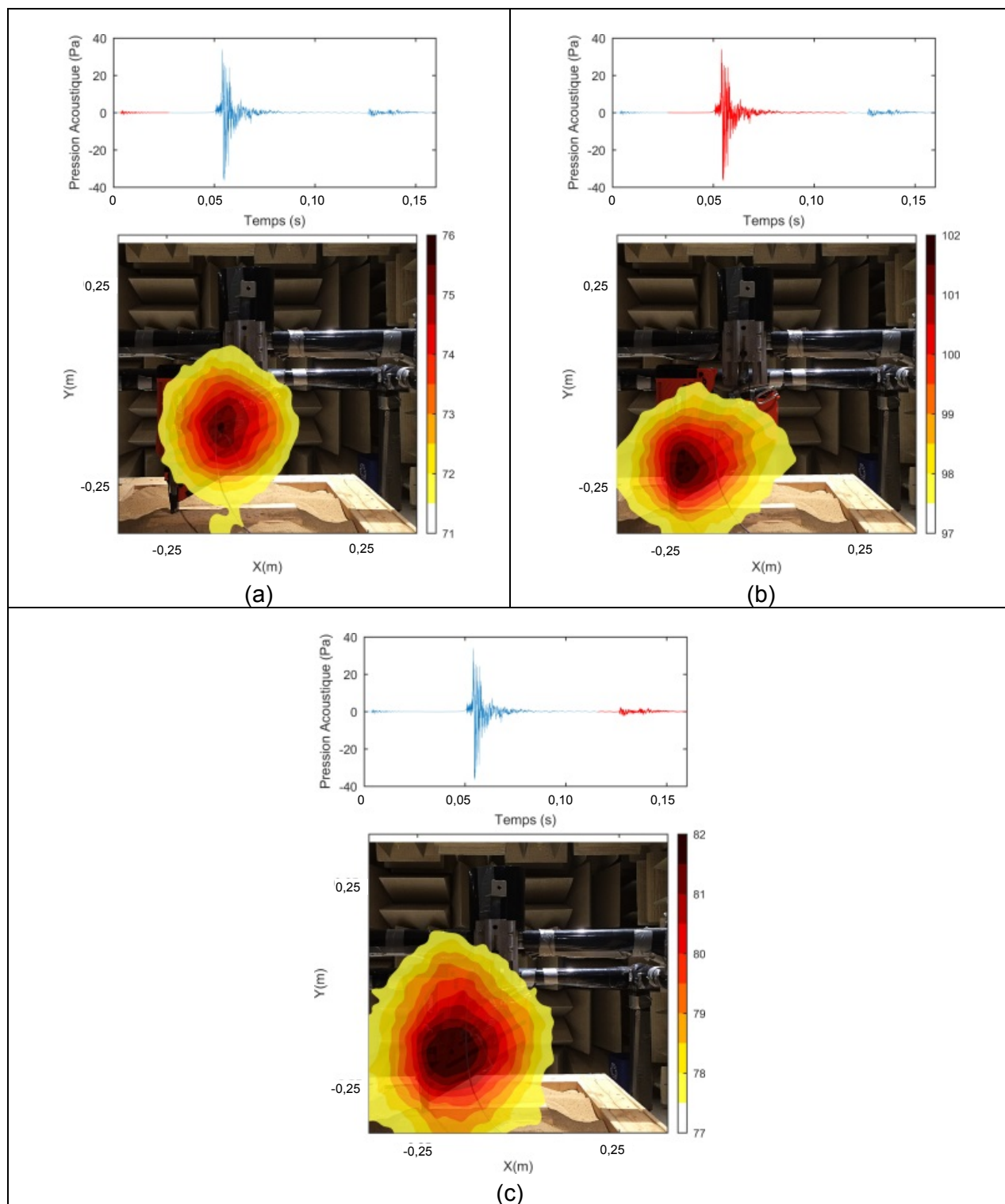
Figure 28 Cartographie des sources acoustiques de la cloueuse à gaz GB1 à 3 instants différents. Les barres de couleur représentent le niveau de pression acoustique en dBA
