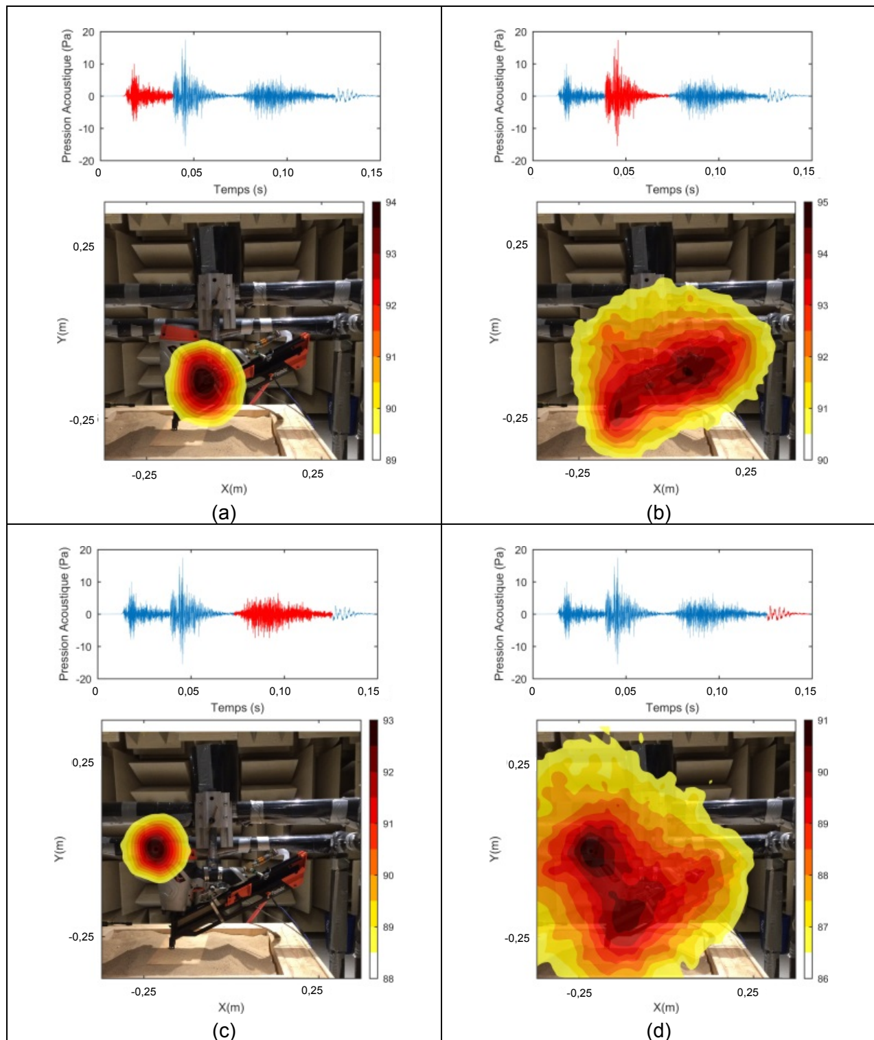
Figure 27 Cartographie des sources acoustiques de la cloueuse pneumatique PB3 à 4 instants différents. Les barres de couleur représentent le niveau de pression acoustique en dBA
