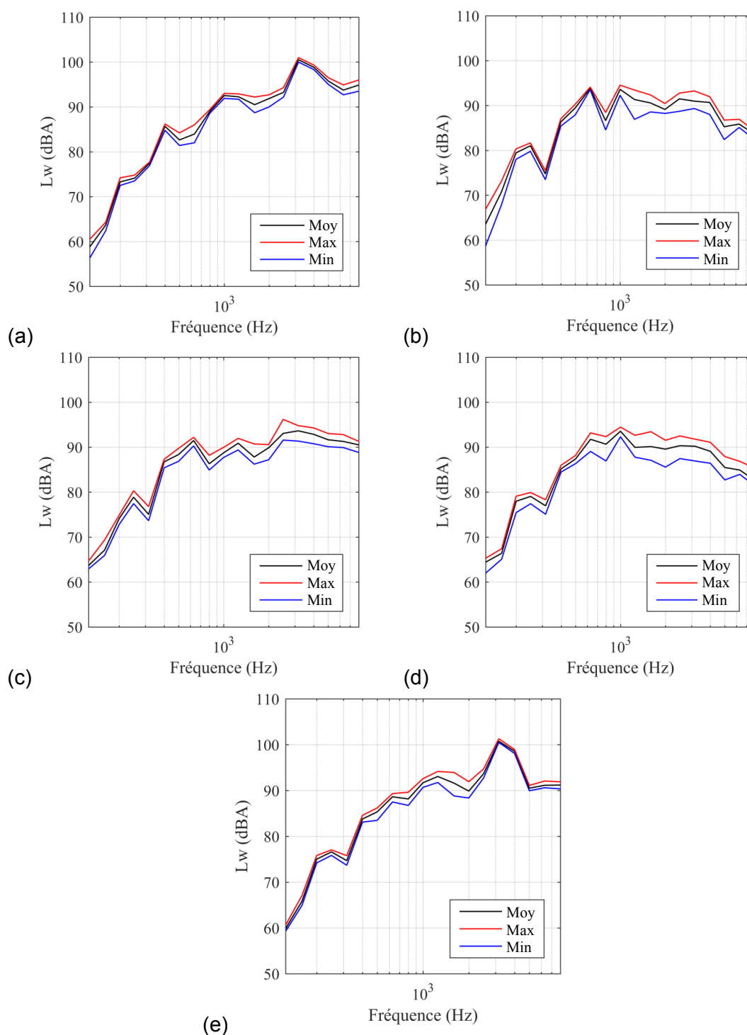
Figure 23 Spectre de puissance acoustique en tiers d'octave pour la cloueuse PB3 : (a) sans traitement, (b) bruit résiduel, (c) bruit de l'échappement d'air, (d) bruit de la pièce travaillée et (e) bruit du corps de la cloueuse
