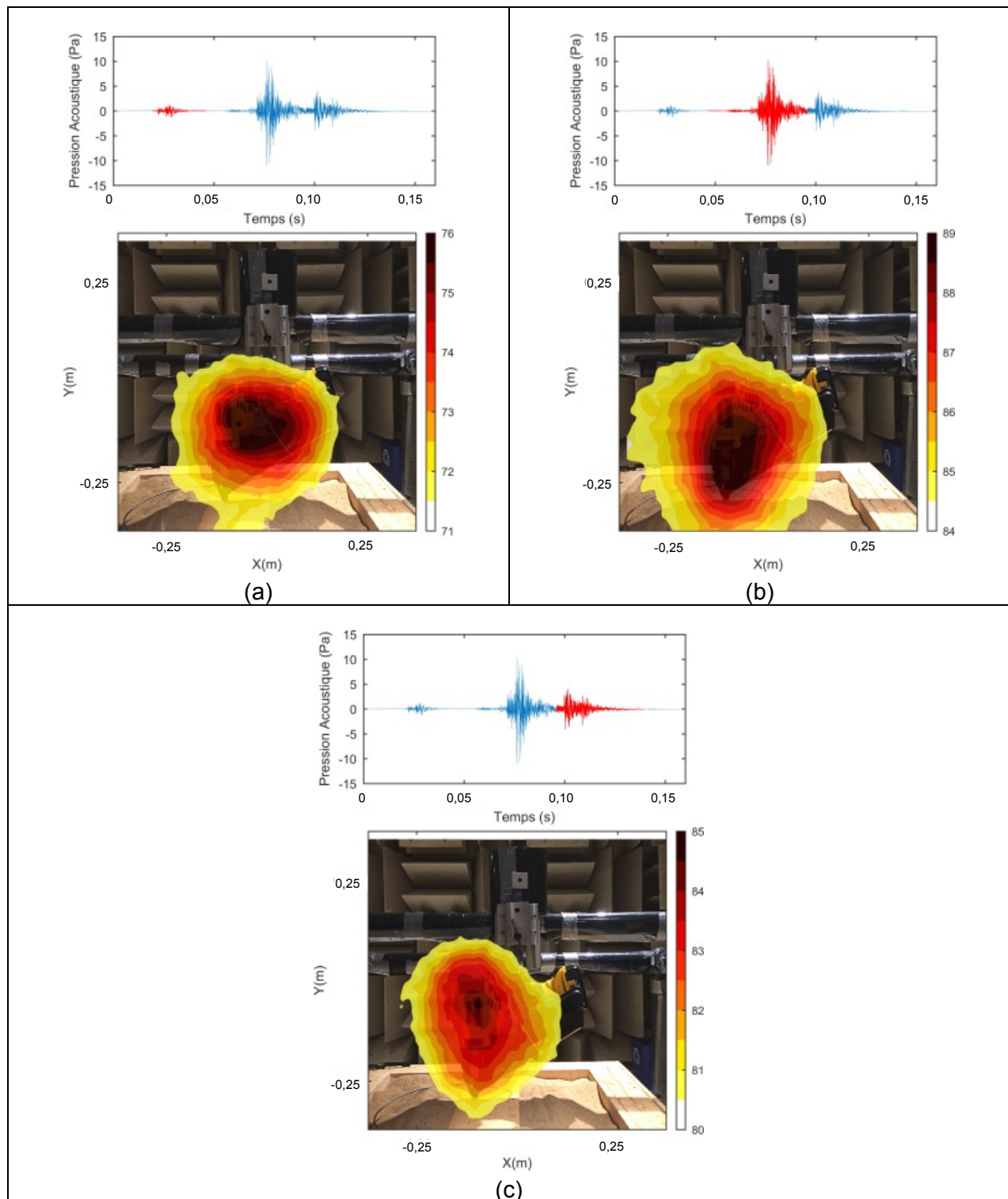
Figure 29 Cartographie des sources acoustiques de la cloueuse électrique EB1 à 3 instants différents. Les barres de couleur représentent le niveau de pression acoustique en dBA
