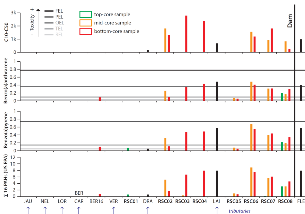
Figure 5. Transect illustrant les concentrations en polluants organiques (C10-C50, benzo(a)anthracène, benzo(a)pyrène et somme des 16 HAPs inclus dans le programme de surveillance de l'Agence pour la Protection de l'Environnement des Etats-Unis (US EPA), en ppm ou mg.kg -1 ) des échantillons de surface (barres noires) et des échantillons issus des carottes courtes (barres de couleur) sur un schéma amont-aval. Les flèches bleues indiquent la jonction avec les affluents de la rivière Saint-Charles.
