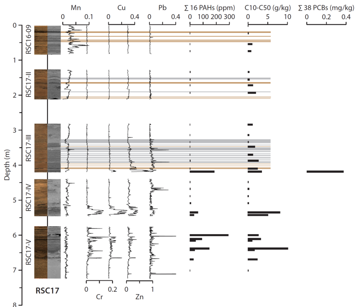
Figure 7. Synthèse des données ITRAX relative aux métaux et des données relatives aux polluants organiques (Somme des 16 HAPs, C10-C50 et somme des 38 congénères BPCs). Les barres horizontales de couleur grise et marron représentent respectivement les dépôts de crues de nature minérale et organique.
