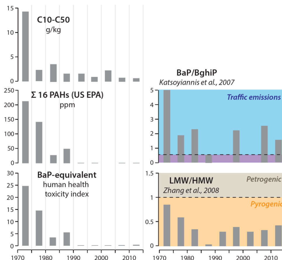
Figure 10. Évolution de la pollution aux composés organiques au cours du temps (gauche). Évolution des sources des HAPs selon différents ratios moléculaires.
