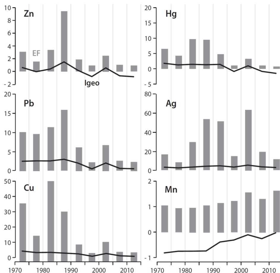
Figure 9. Évolution des facteurs d'enrichissement (EF) et des indices de géo-accumulation (Igeo) depuis la construction du barrage dans les sédiments de la carotte RSC17. Zn : zinc - Pb : plomb - Cu : cuivre - Hg : mercure - Ag : argent - Mn : manganèse.
