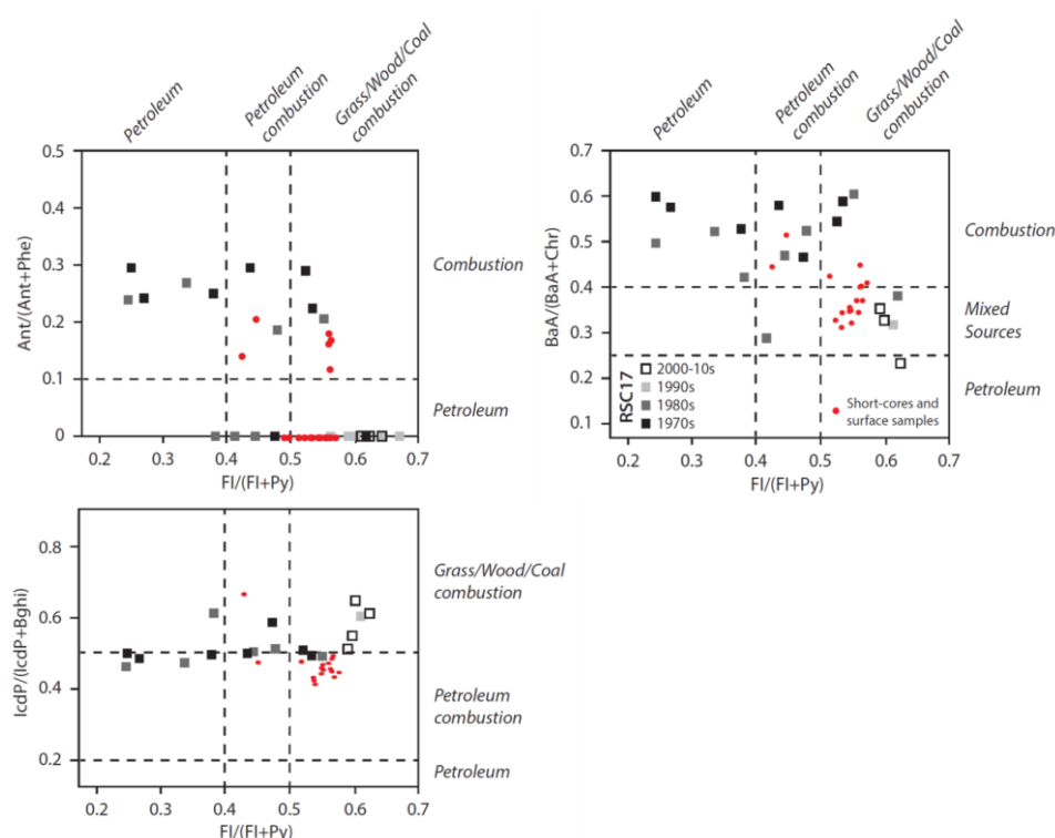
Figure 11. Ratios illustrant les possibles origines pétrogénique et pyrogénique (combustion d'essence, de charbon et de bois) des HAPs dans les sédiments de la rivière Saint-Charles.
