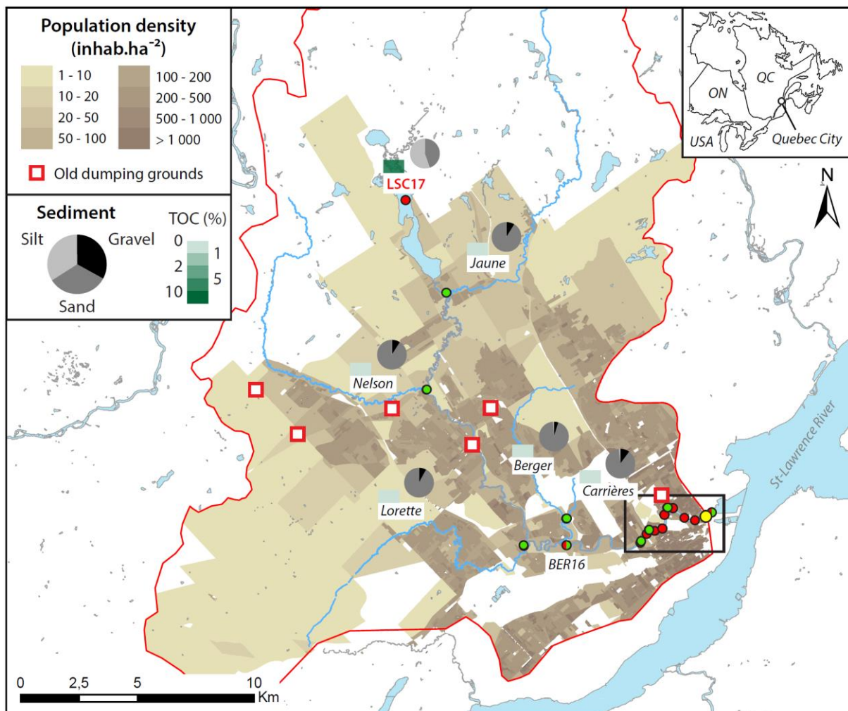
Figure 2. Carte indiquant les résultats des analyses granulométriques (diagramme camembert) de la teneur en COT (carré vert) pour les différents échantillons de surface localisés dans la partie amont du bassin versant. L'encart en noir correspond au secteur aval de la rivière présenté dans la Figure 3.
