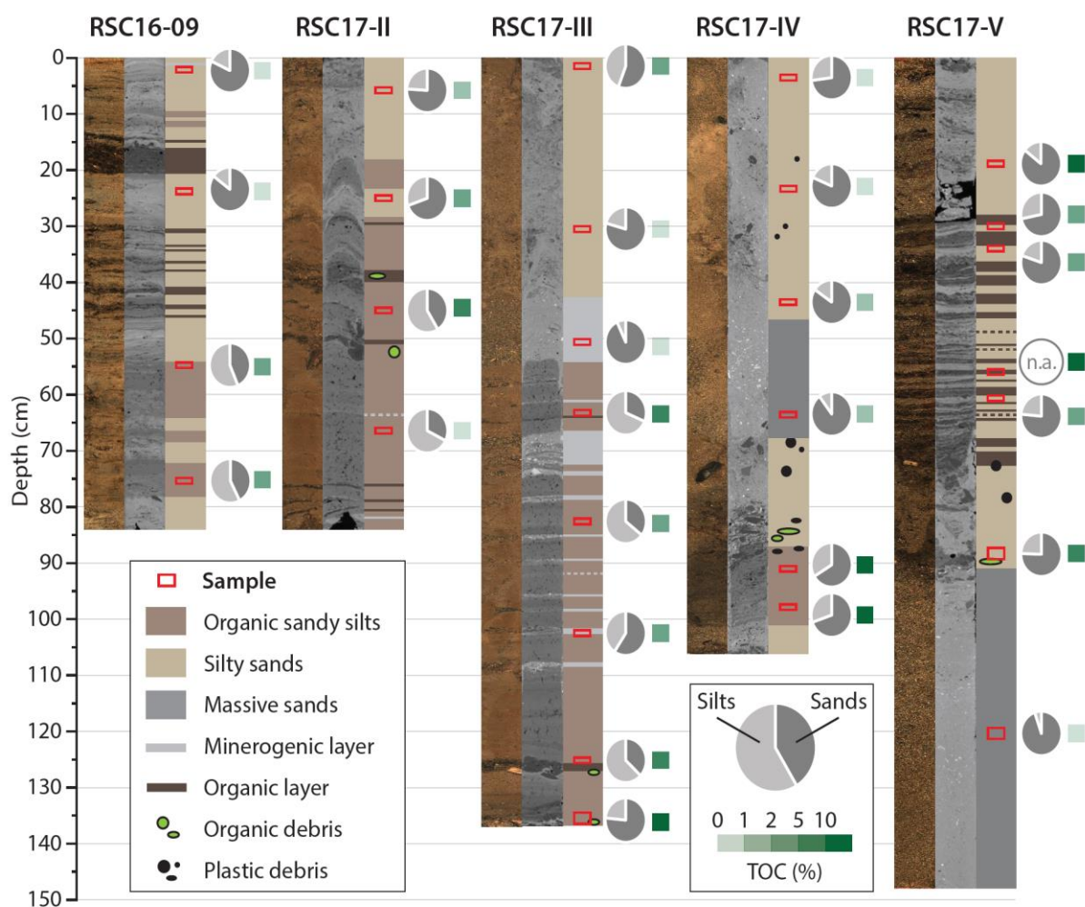
Figure 6. Images numériques et radiographiques des cinq sections de tubes utilisées pour reconstruire la grande carotte composite RSC17. Les analyses ponctuelles (COT et granulométrie) sont représentées de la même manière que sur les figures précédentes. Ces analyses ont permis de définir les faciès sédimentaires synthétisés à travers le log apposé à droite de chaque section.
