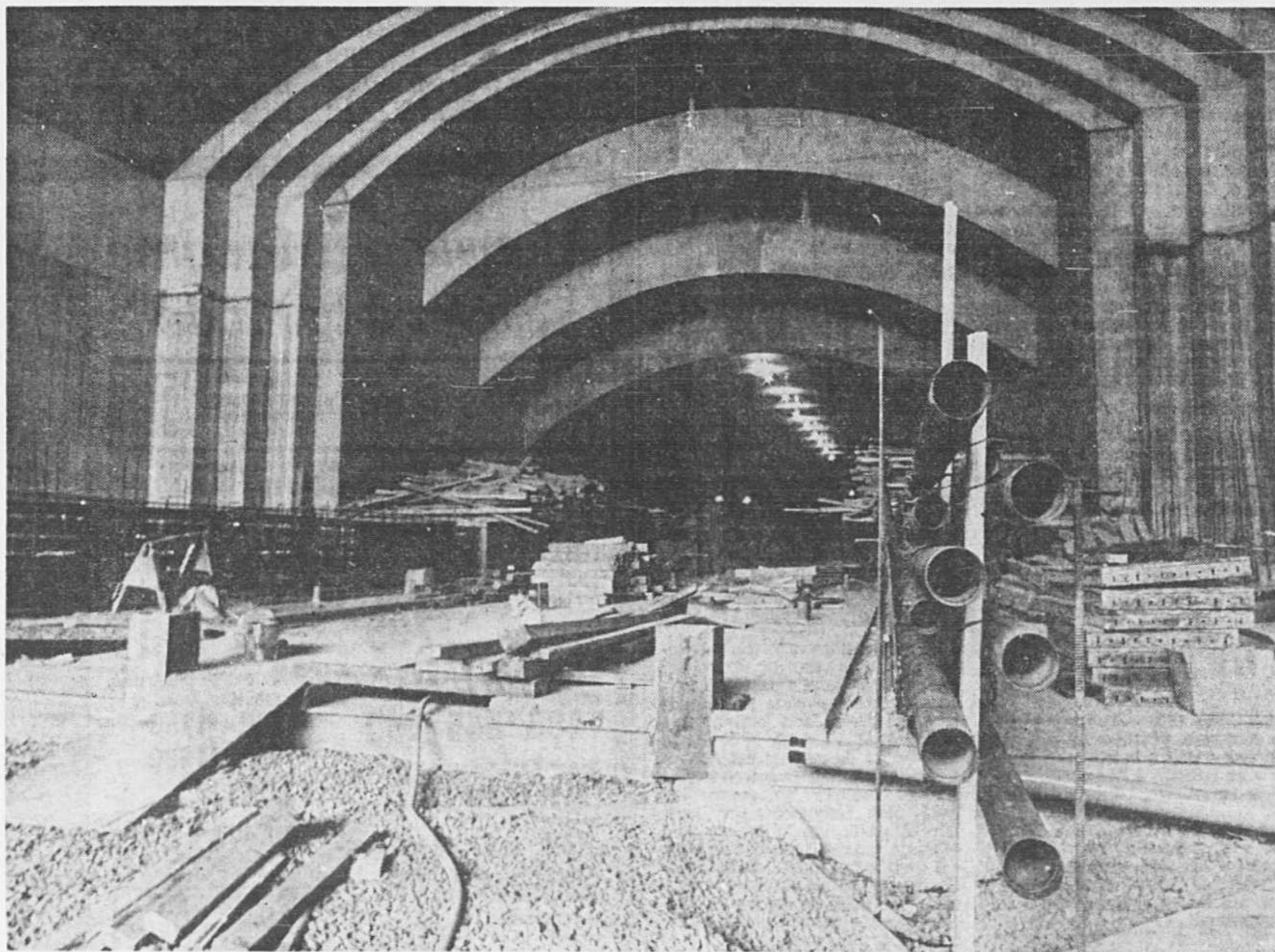
Le gros-oeuvre de la station Langelier est presque terminé. A la droite de la photo, on aperçoit les conduits utilisés pour les câbles électriques, qui seront enfouis dans le ciment, comme le recommandait le rapport Tellier par mesure de sécurité.
