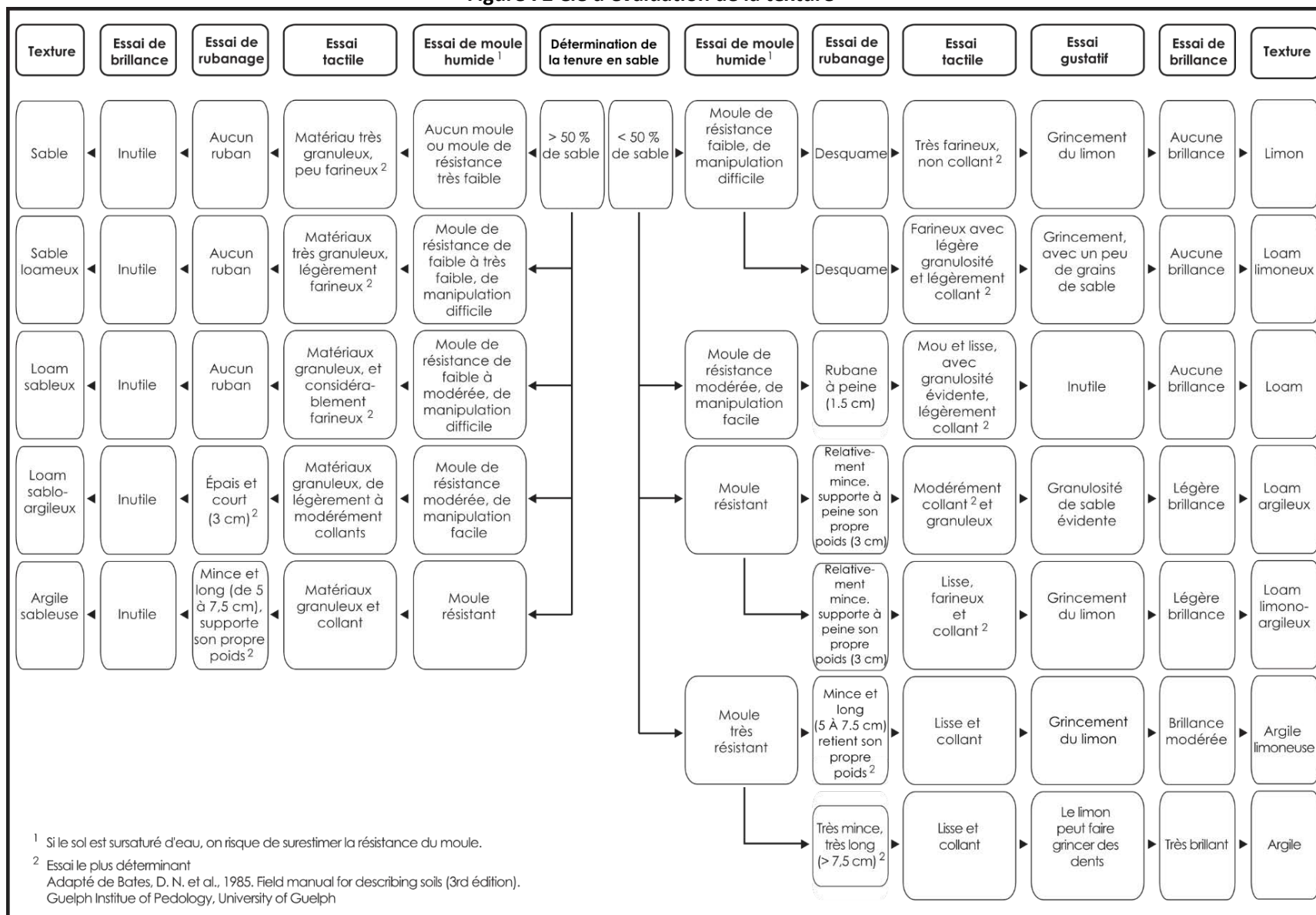
Figure 72 Clé d'évaluation de la texture
