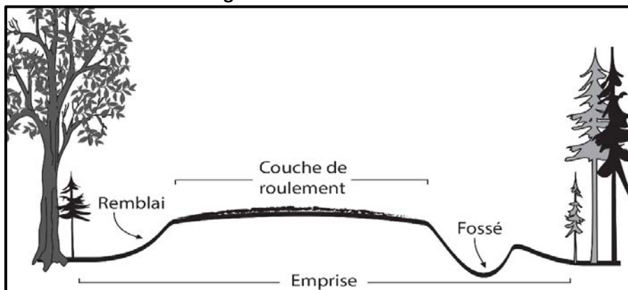
Figure 12 Profil de chemin
