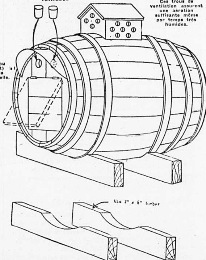
Bouchons de liège pour fermer, au besoin, les trous de ventilation
