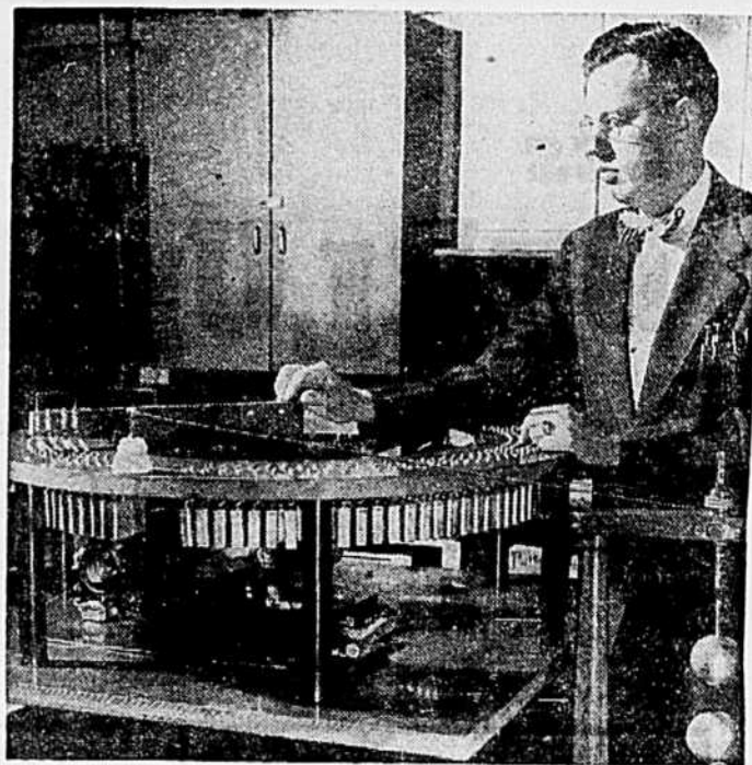
UN MULTIPLICATEUR DE VOLTAGE. — Un ingénieur de Schenectady, New-York, se prépare à expérimenter une nouvelle machine appelée "multiplicateur de voltage". Cette machine a été conçue pour multiplier le voltage de 100 volts d'un petit générateur en un voltage total de 100,000 volts. Cette machine qui n'en est encore qu'à la période d'expérimentation, aux laboratoires de la General Electric, pourra être utilisée, ultérieurement, pour le fonctionnement d'appareils à Rayons X ou de briseurs d'atomes.
