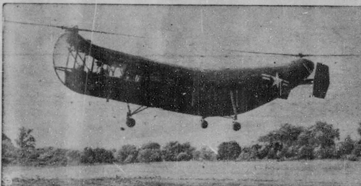
Avec une hélice évoluant au sommet de chacune de ses extrémités, le nouvel hélicoptère HRP-1 fait une envolée d'essai. Il est pourvu d'un moteur de 600 chevaux-vapeur et peut atteindre une vitesse de 100 milles à l'heure, monter et descendre verticalement avec une charge de plus d'une tonne. Les essais se font au centre naval d'essais aériens de Patuxent, Maryland. Vingt de ces transports aériens ont été commandés par la marine.
