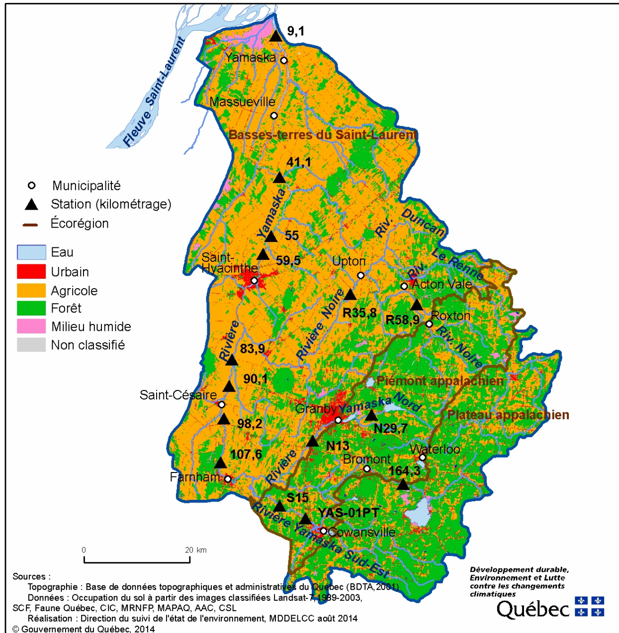
Figure 1 Localisation des stations d'échantillonnage des poissons des rivières Yamaska, Yamaska Nord, Yamaska Sud-Est et Noire
