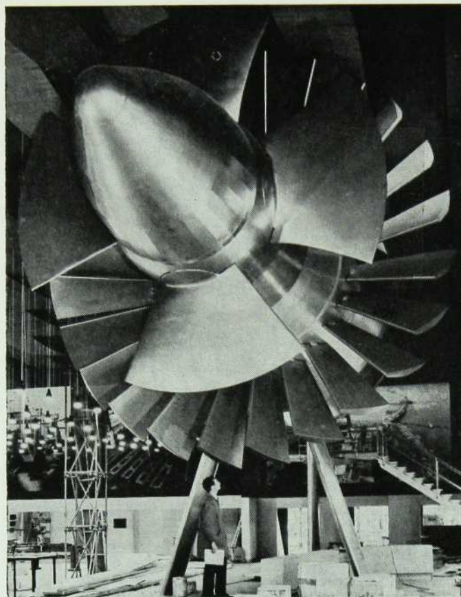
Générateur destiné à équiper les centrales marémotrices de France.
