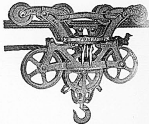
CHARIOT À FOIN "JUTRAS"
