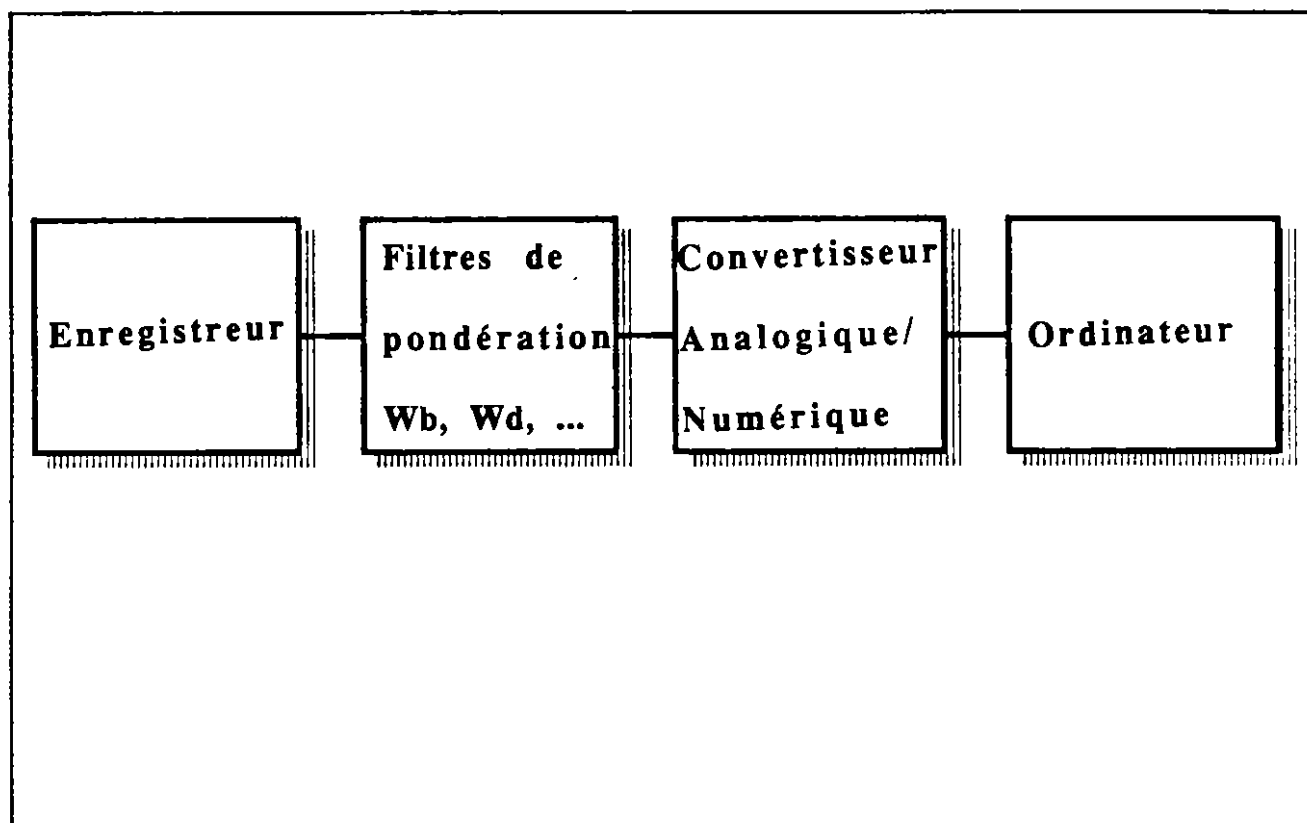
Figure 4: Montage expérimental pour l'évaluation des accélérations RMS et RMQ et du facteur de crête.
