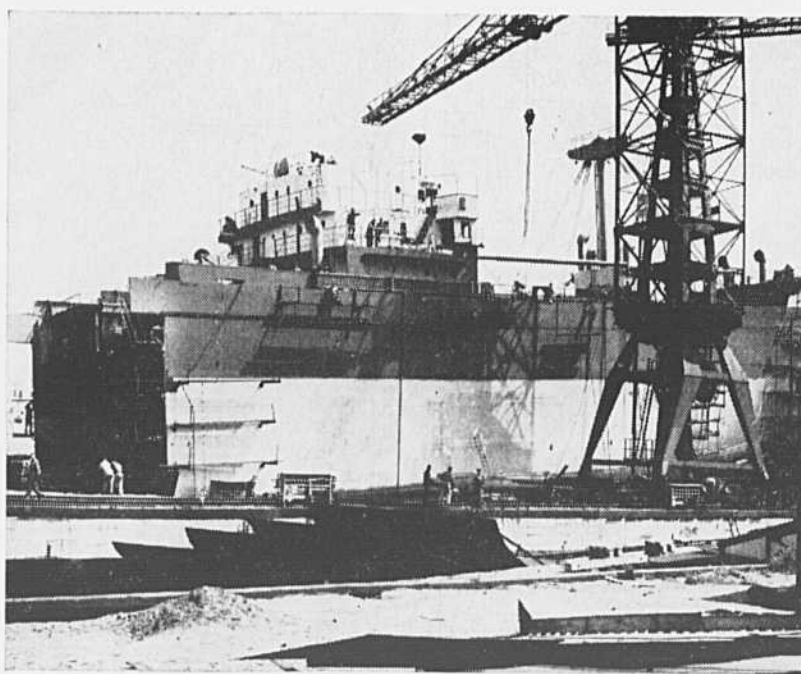
Aux chantiers maritimes de Bolnes, près de Rotterdam, Hollande, va être lancé prochainement un demi-bateau. Il s'agit de la partie-avant du navire suisse Nyon qui s'échoua en novembre 1958 sur la côte d'Ecosse. La poupe ne subit pas trop d'avaries et put être dégagée et remise à neuf. Les autorités passèrent alors commande aux chantiers de Hollande pour la construction de la proue d'un navire de tout point identique à la précédente et les deux moitiés seront soudées pour ensuite reprendre la mer sous le nom de Nyon-II .
