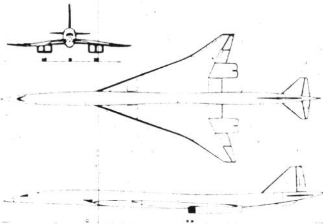
Un supersonique silencieux, muni de cinq réacteurs, projet de la McDonnell Douglas.
