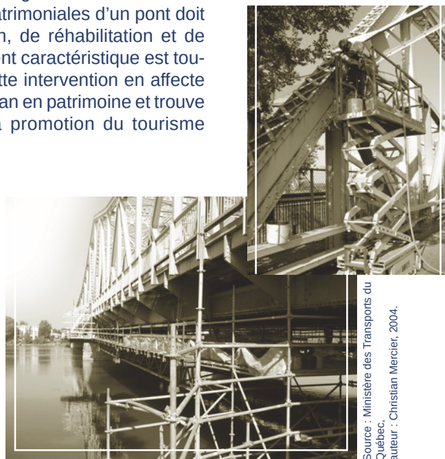
IPS de 93 : Travaux de conservation en 2004 au pont Lachapelle sur la route 117 Nord à Laval. Structure métallique à sous-système Waddell's « A » construite par encorbellement par la Dominion Bridge en 1930.
