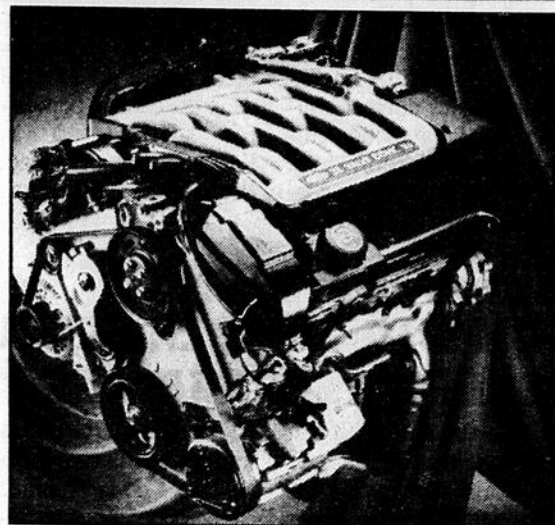
Ce V8 multisoupapes s'allume avec des bougies "platine" qui ne seront remplacées que lorsque l'odmètre aura atteint 100 000 kilomètres. Heureusement, elles sont difficilement accessibles.
