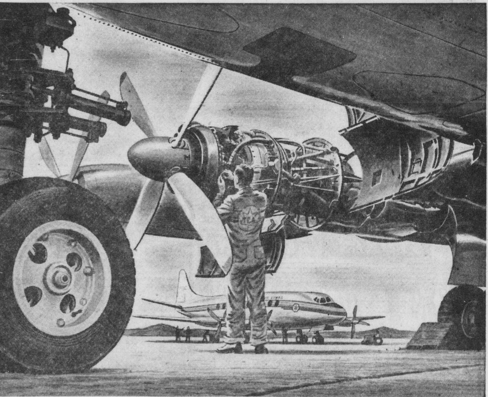
Les 4 moteurs Rolls-Royce "Dart" du quadrimoteur Viscount Vickers-Armstrongs développent, au total, 5600 CV (environ 1 CV par 10 onces de poids des moteurs) plus une poussée de 1460 lb fournie par les gaz d'échappement. Le "Dart" est un moteur à turbo-propulsion dont aucune pièce n'a de mouvements alternatifs et qui, actionnant une hélice à vitesse relativement basse, est d'un fonctionnement exceptionnellement peu bruyant.
