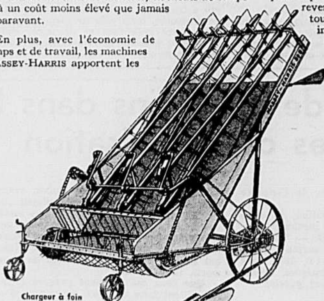
Chargeur à foin Massey-Harris No 8
