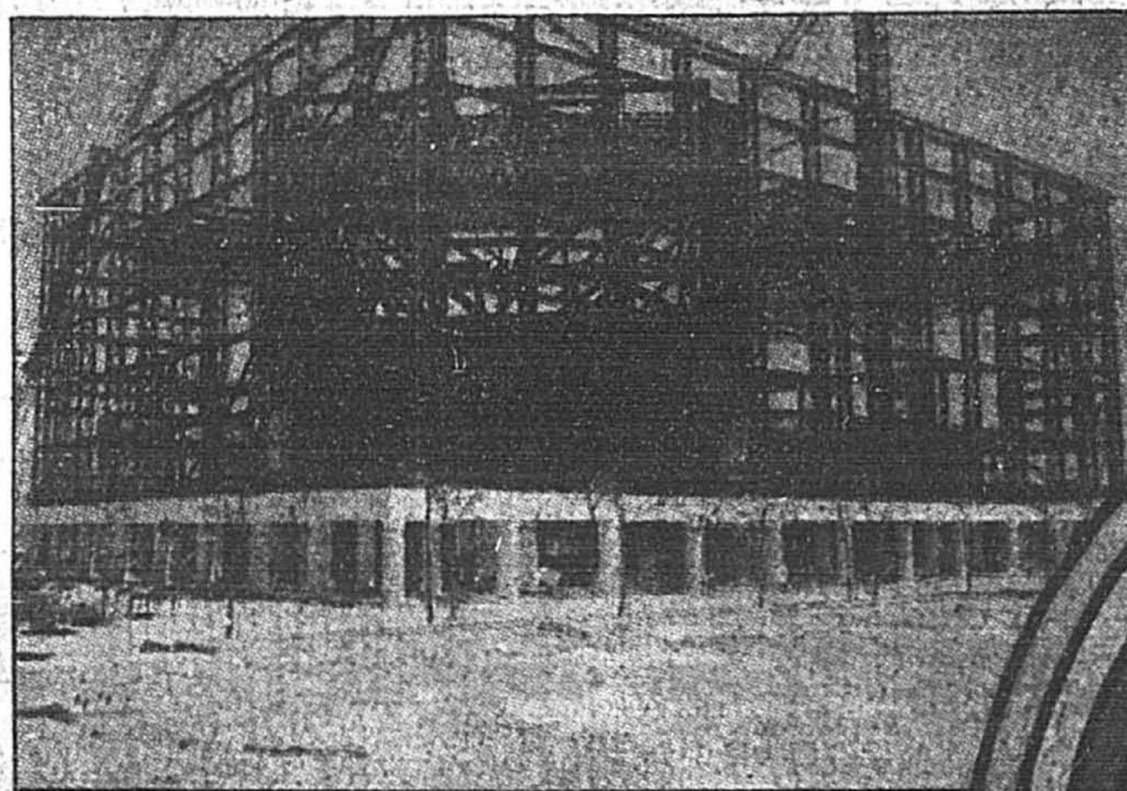
Ci-dessus, la structure imposante du pavillon canadien en construction dans l'île de la Chartreuse.
