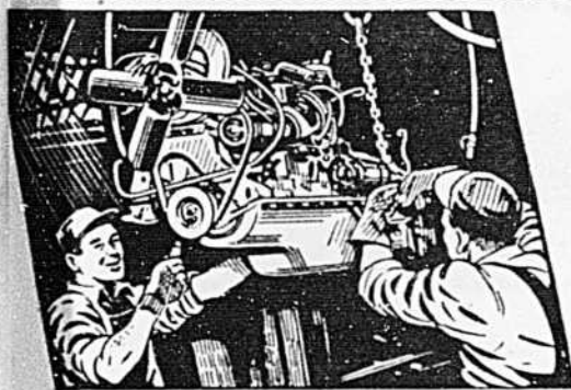
Des transporteurs aériens actionnés par électricité déposent les moteurs Dodge, de fabrication canadienne aussi, sur les armoires. C'est le départ.
