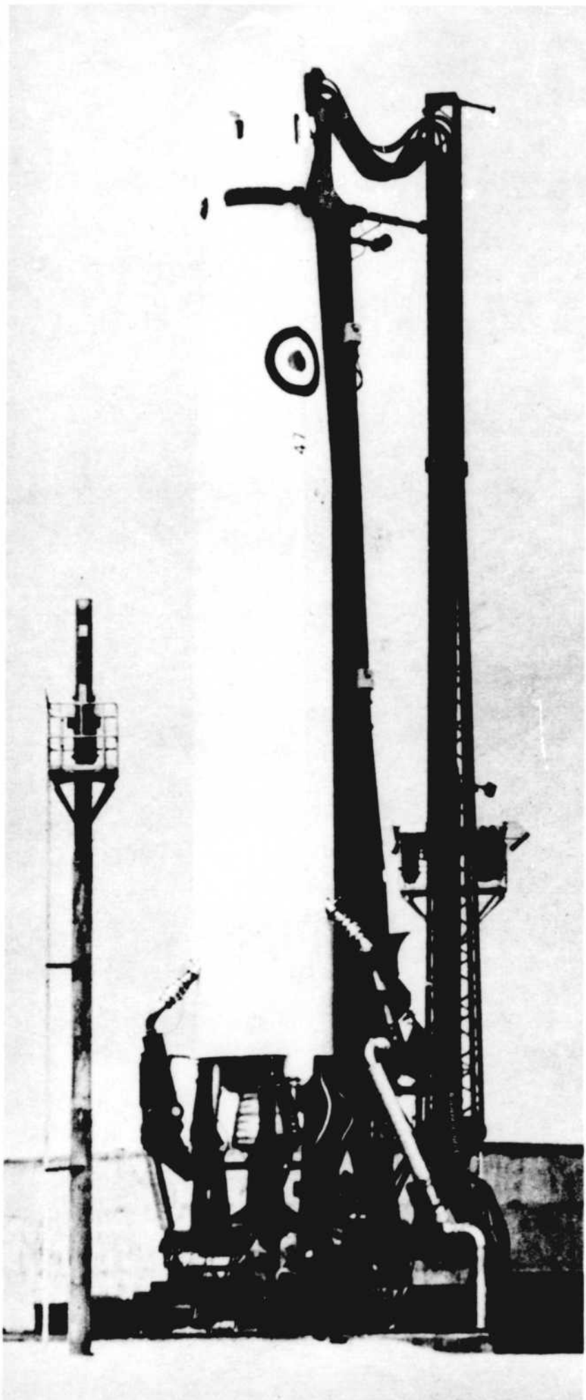
Une fusée Thor en position de départ. Les servants de l'engin semblent des nains à côté de l'énorme cylindre. Pesant 110,000 livres, ce missile a une portée de 1,700 milles.
