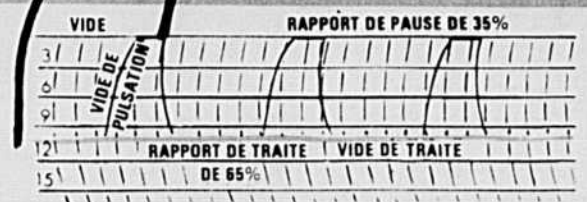
Les graphiques ci-dessus de comparaison de la stabilité du vide indiquent le vide stable de ZERO CONCORD en comparaison d'un système à vide qui fluctue. La ligne rouge du graphique de droite ci-dessus révèle comment fluctue le vide d'un système ordinaire, vu qu'on traite les vaches et qu'on achemine
