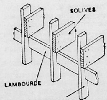
LAMBOURDE
