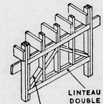
PIED-DROIT
