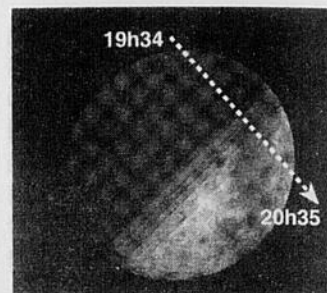
L'occultation de Saturne par la Lune le 20 février 2002, vue de Montréal. Sur ce dessin, la Lune se déplace vers le haut et vers la gauche par rapport au reste de la voûte céleste. La planète Saturne semble alors bouger dans l'autre sens, comme l'indique la flèche, et passe derrière la Lune (tirets).
