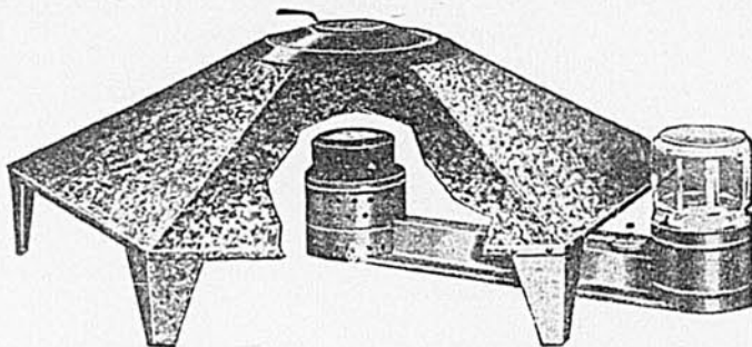
ELEVEUSE BUCKEYE A FLAMME BLEUE — Cette éleveuse à l'huile peut être employée sans crainte et assure la chaleur nécessaire à la protection de vos poulets. Elle est la meilleure valeur jamais offerte dans les éleveuses à l'huile.
