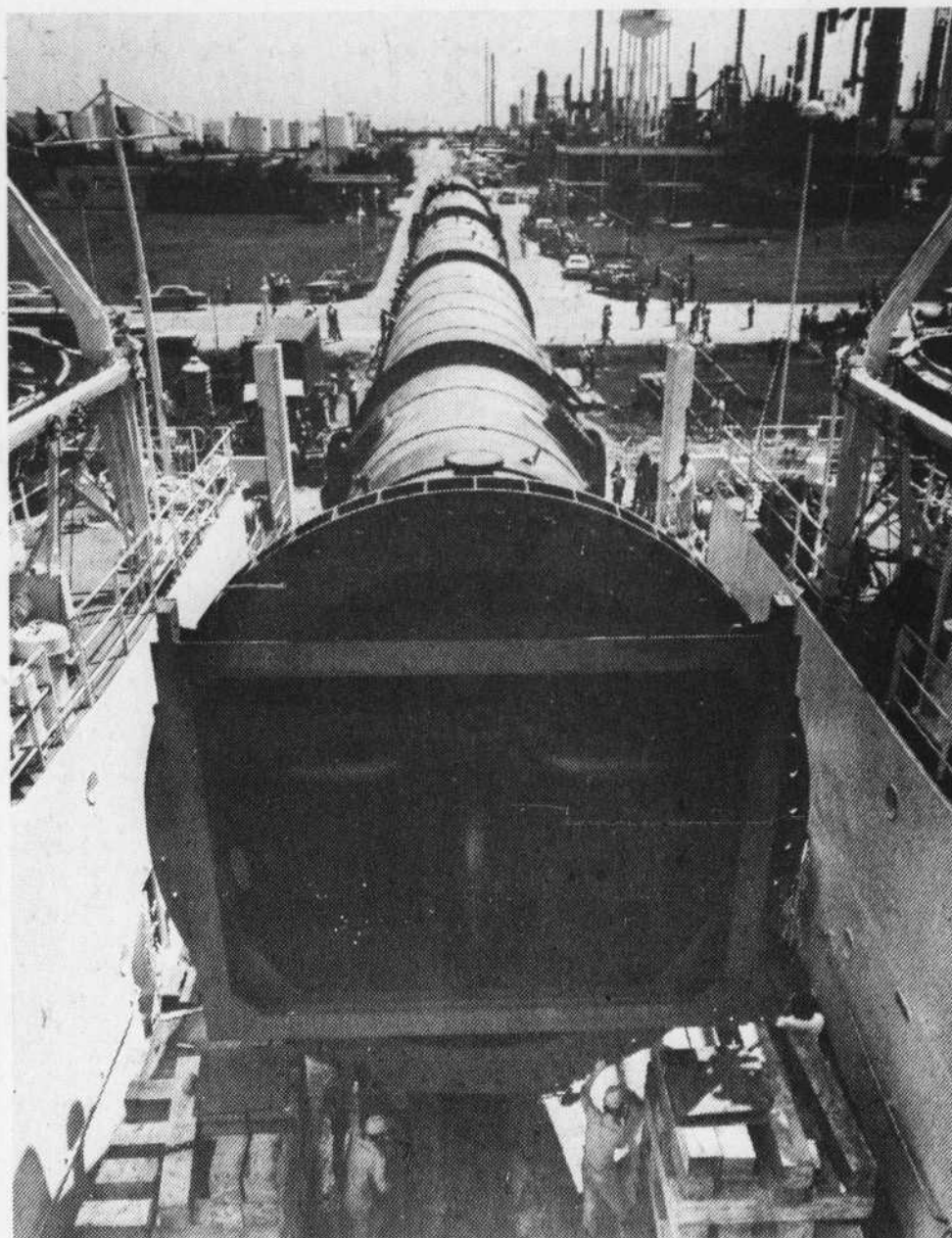
La plus haute tour préfabriquée du Canada termine le voyage de 4,000 milles qui l'a conduite des Pays-Bas à la raffinerie de Shell Canada à Sarnia en Ontario. La tour, qui pèse 455 tonnes, dominera de ses 266 pieds la nouvelle usine de polypropylène de Shell présentement en construction.
