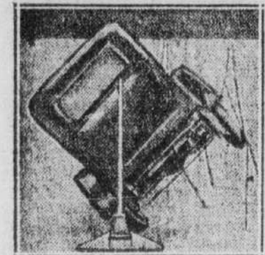
Vignette No 1. — Avant de manifester une tendance à se renverser, la voiture fermée doit pouvoir être redressée de 52 degrés.
