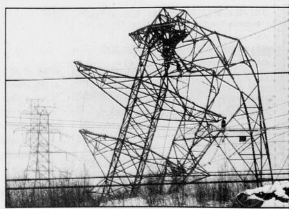
Quatre pylônes de transmission se sont affaissés à Dartmouth.
