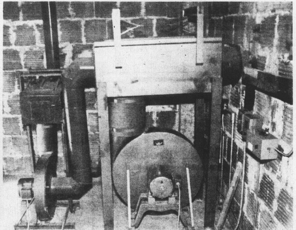
La salle des machines de l'orgue. Deux énormes moteurs soufflant comme quelques milliers de poumons.
